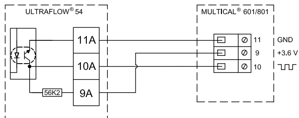
Схема 1 – Соединение трехжильным кабелем, MULTICAL® 602/801 через выходной модуль (Y=2). Длина кабеля до 25 метров.
